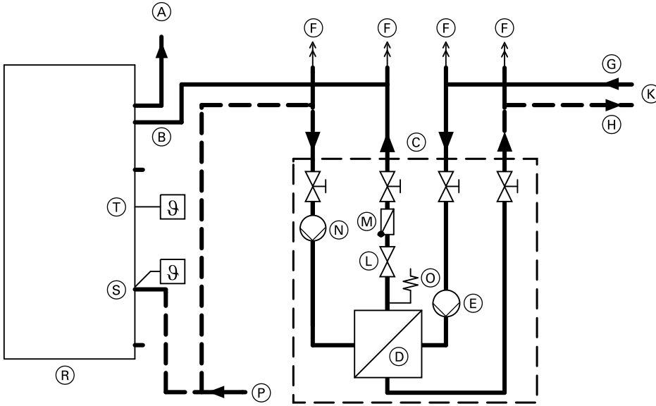
Sabit gidiş suyu sıcaklığında işletme
