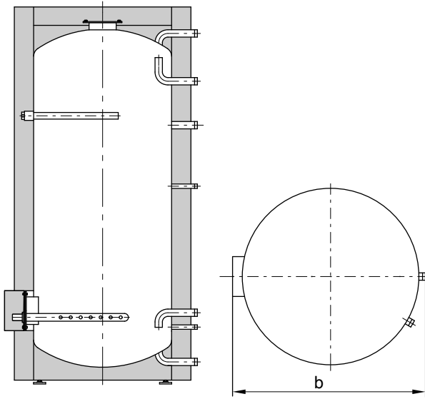
Besleme lanslı Vitocell 100-L
