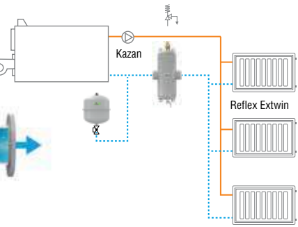
Extwin "Çelik" sistemi birleşik mikro kabarcık, tortu ve pislik ayırma şeması
