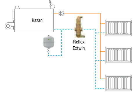
Extwin "piring" sistemi birleşik mikro kabarcık, tortu ve pislik ayırma şeması
