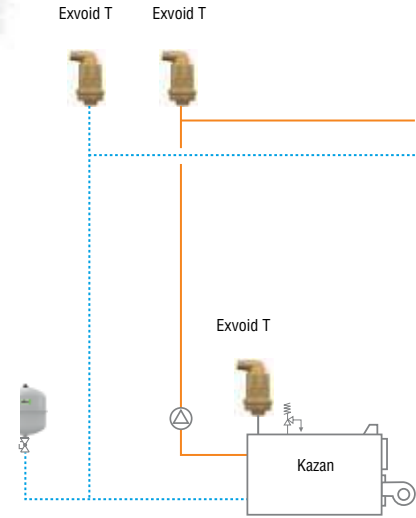
Exvoid T sistem için hava tahliye şeması
