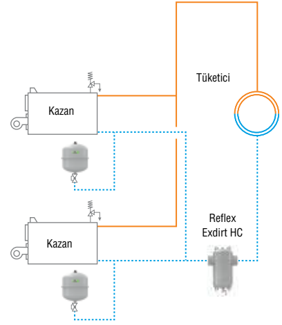
Exdirt "çelik" HiCap sistem için tortu ve pislik ayırma şeması
