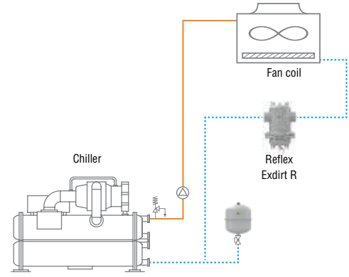
Exdirt "çelik" sistem için tortu ve pislik ayırma şeması
