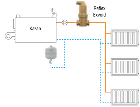
Exvoid "pining" sistem için hava tahliye şeması
