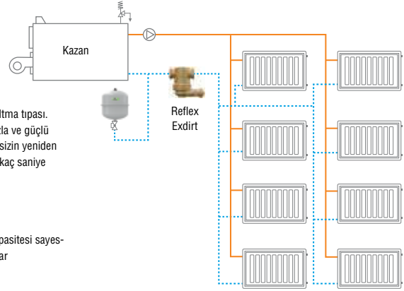
Exdirt "piring" sistem için tortu ve pislik ayırma şeması
